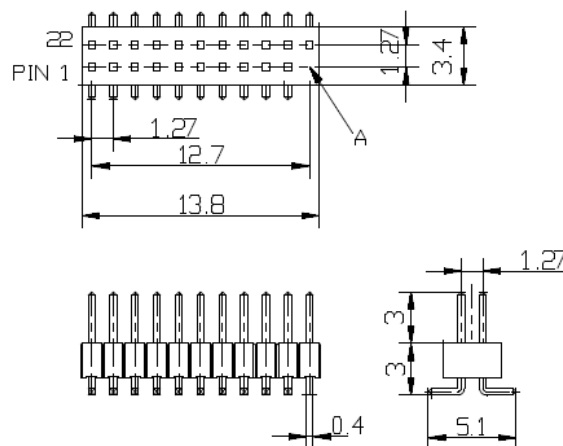
Figura 3: barra de pinchos típica, A = posición del pin índice (evita-errores)
