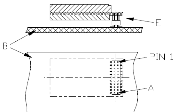
Figura 5: Variante vuelta A = posición del Pin 11 evita-errores B = placa del vehículo C = espacio a dejar libre en la placa E = barrita de pinchos
