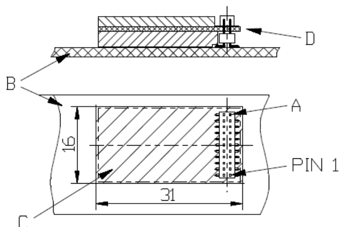
Figura 4: Variante compacta A = posición del Pin 11 evita-errores B = placa del vehículo C = Espacio a dejar libre en la placa D = Placa del descodificador
