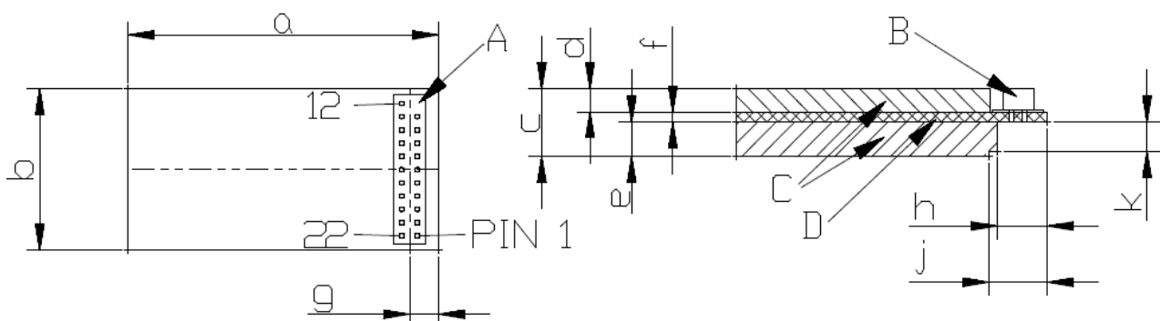
Figura 1: Descodificador visto desde encima, lado de los pinchos de la variante compacta.
