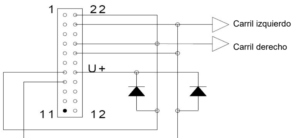
Figura 6: Puenteo típico
