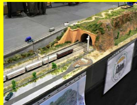
Trens escala N
